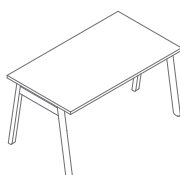
BOB03 1400 / 800 / 740 36.5 kg
