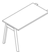
PLB03 600 / 1200 / 740 20.6 kg
