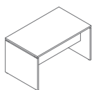
BVG03 1400 / 800 / 740 77.45 kg
