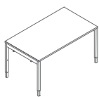
BOY03R 1400 / 800 / 640-860 41.55 kg
