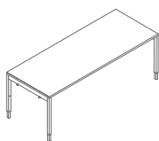
BOY06R 2000 / 800 / 640-860 51.3 kg
