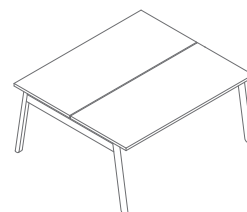
BOB46 1600 / 1410 / 740 75 kg
