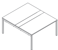
SY04 1400 / 1610 / 740 76.75 kg
