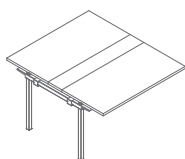
SY32 1200 / 1410 / 740 55 kg
