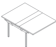
SY12 1200 / 1610 / 740 59.55 kg
